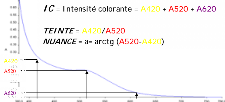
Spectre d'absorption
